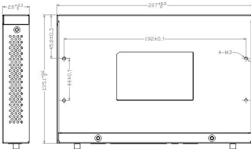
路由器尺寸
