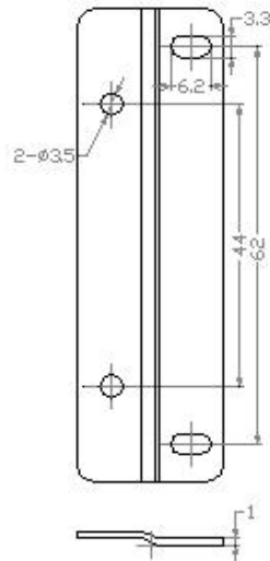
固定片尺寸
