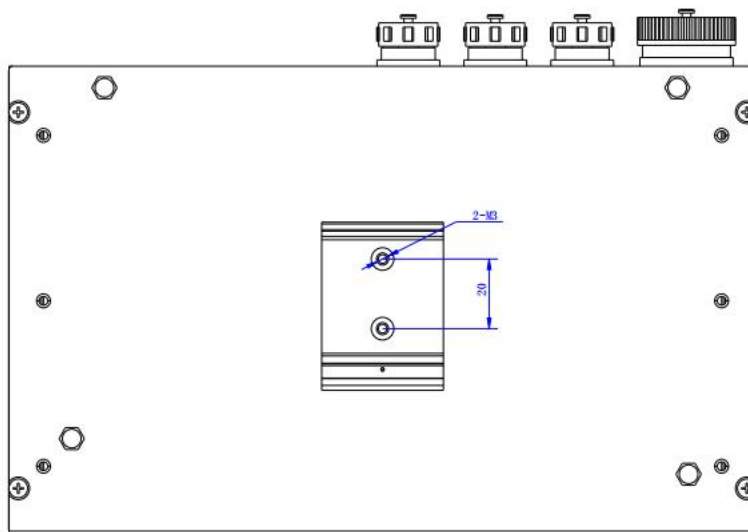
导轨安装示意图
